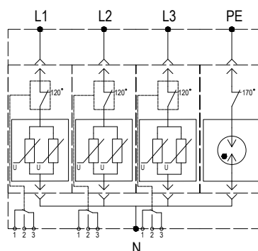
Принципиальная схема
