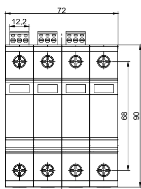
Габаритные размеры
